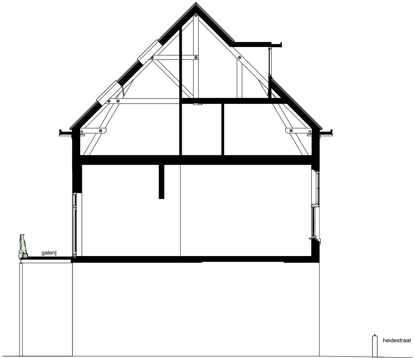
DOORSNEDE
